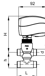
AMV(E) 130/140 + VZ 4
